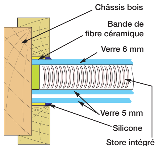
COUPE HORIZONTALE Châssis bois double vitrage PF IH30 CF I/4 H selon P.V. n° 03-V-162
