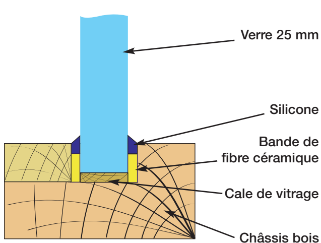
COUPE VERTICALE Châssis bois simple vitrage CF IH PF IH selon P.V. n° 98-V-021
